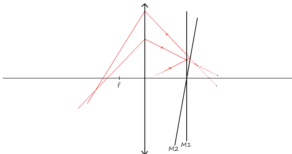
FIGURE 5 – Coin d'air
